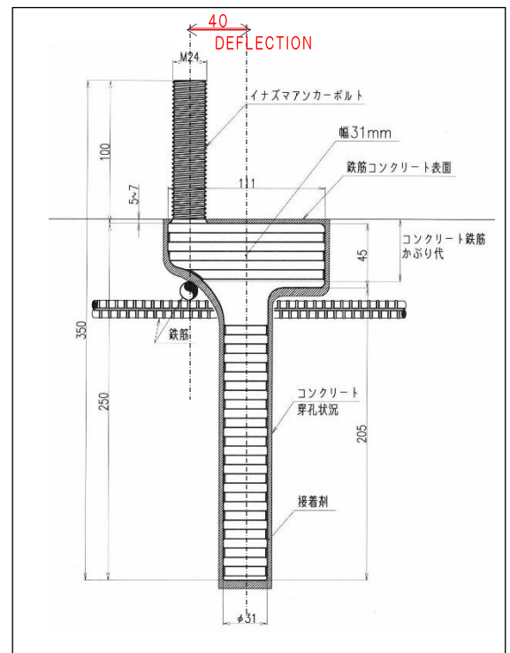
<T22, T24 使用状態図> (取付ねじ部 M22, M24)
