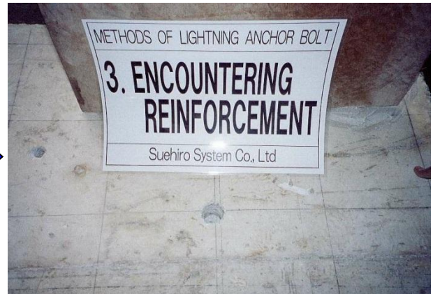
<穿孔位置に鉄筋干渉>
